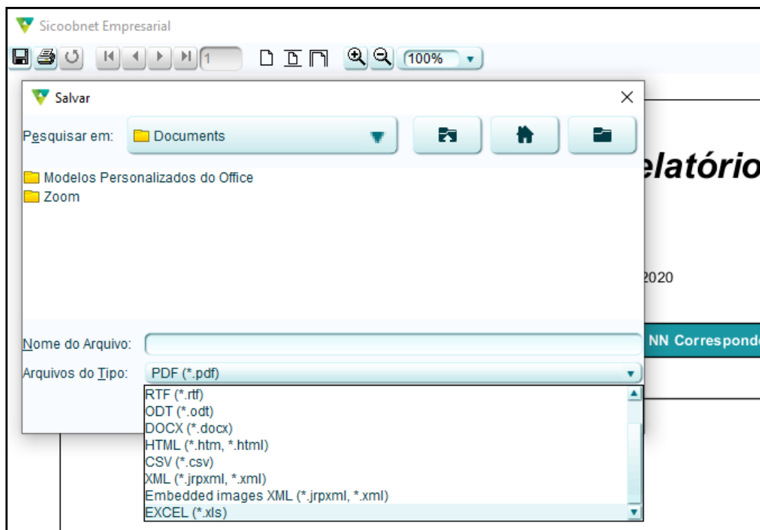
Figura 5 - Salvar relatório
