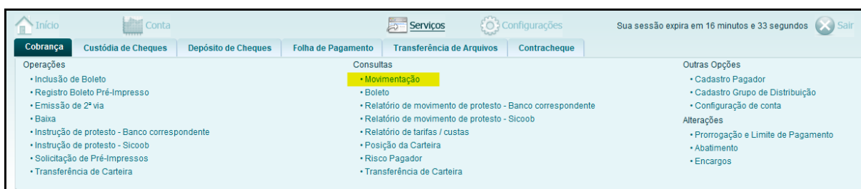
Figura 1 - Menu Cobrança
