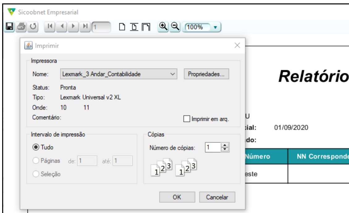
Figura 6 - Imprimir relatório
